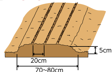
トンネル被覆（穴開きフィルム）【図2】
